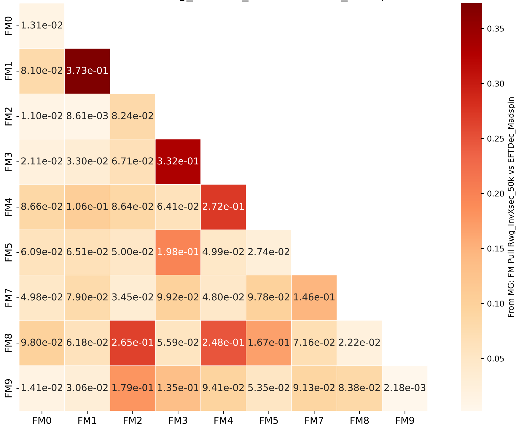
From MG: FM Pull Rwg_InvXsec_50k vs EFTDec_Madspin
