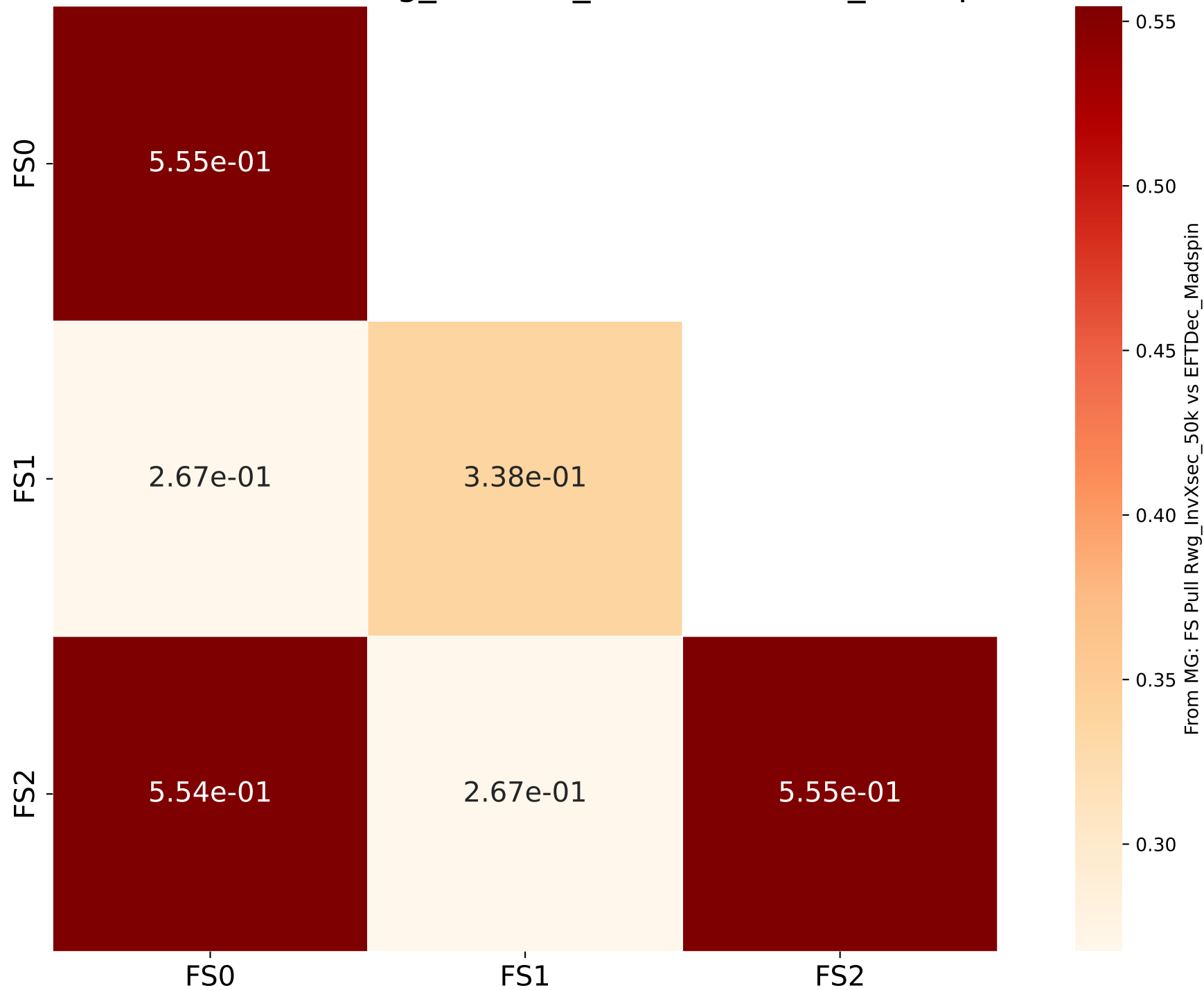
From MG: FS Pull Rwg_InvXsec_50k vs EFTDec_Madspin
