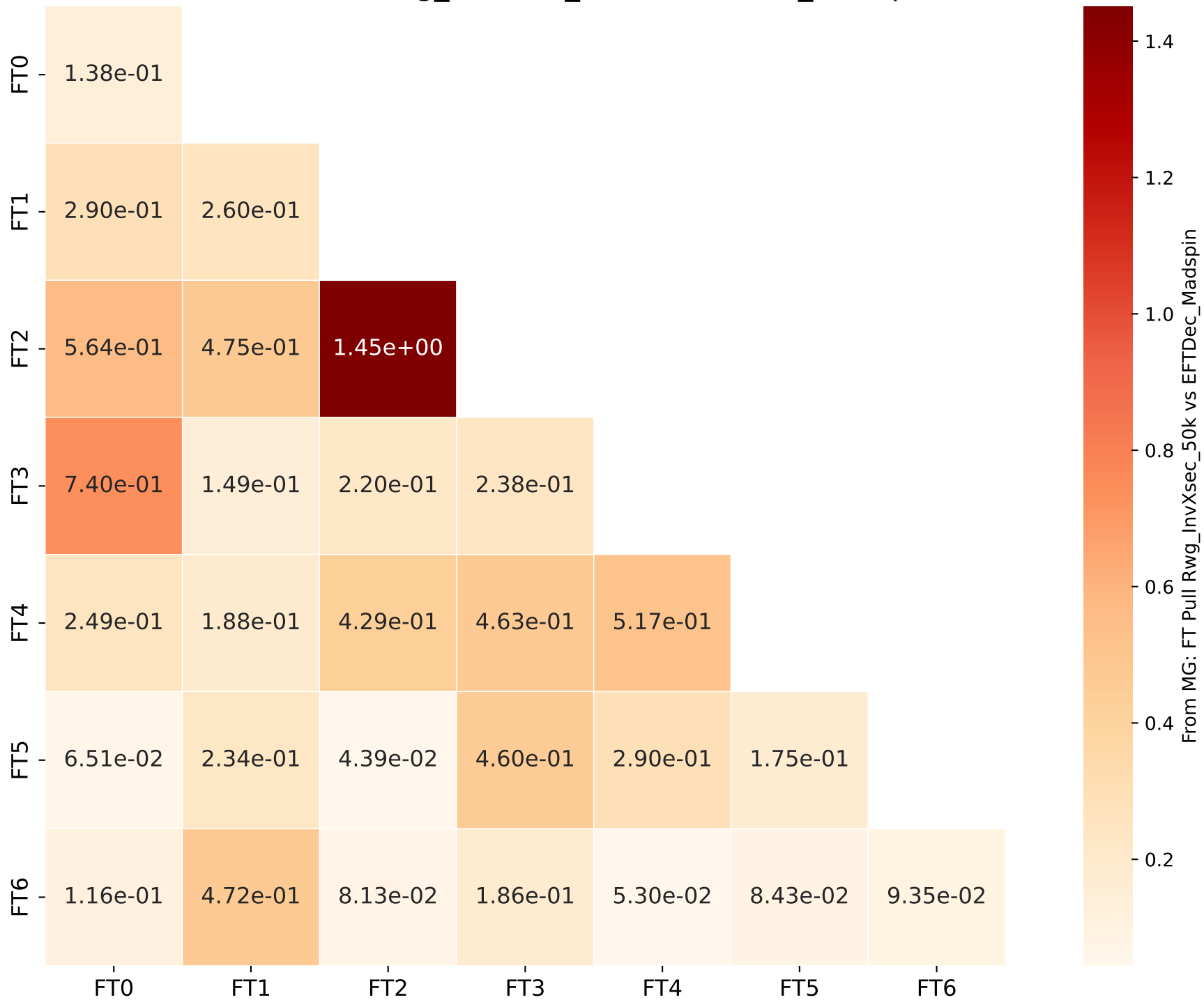
From MG: FT Pull Rwg_InvXsec_50k vs EFTDec_Madspin
