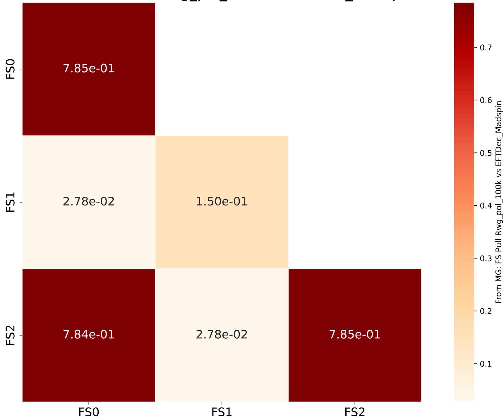
From MG: FS Pull Rwg_pol_100k vs EFTDec_Madspin
