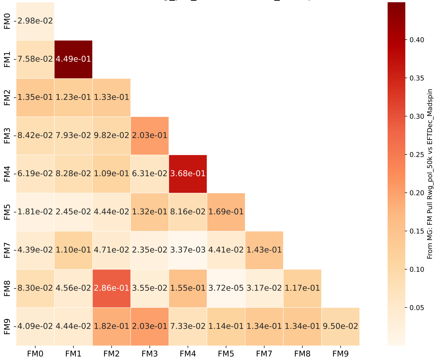
From MG: FM Pull Rwg_pol_50k vs EFTDec_Madspin
