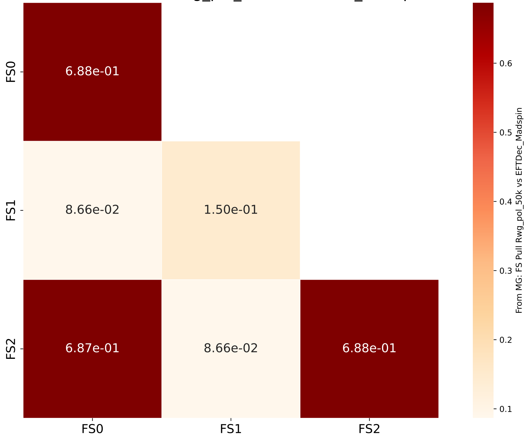
From MG: FS Pull Rwg_pol_50k vs EFTDec_Madspin
