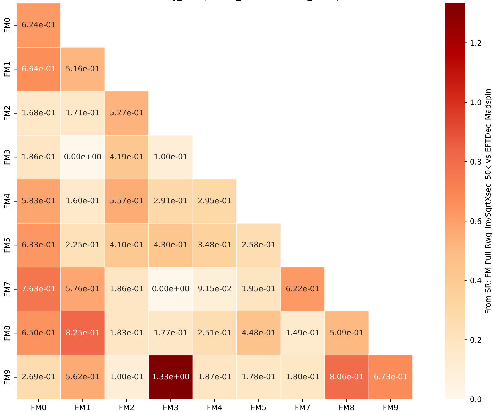
From SR: FM Pull Rwg_InvSqrtXsec_50k vs EFTDec_Madspin
