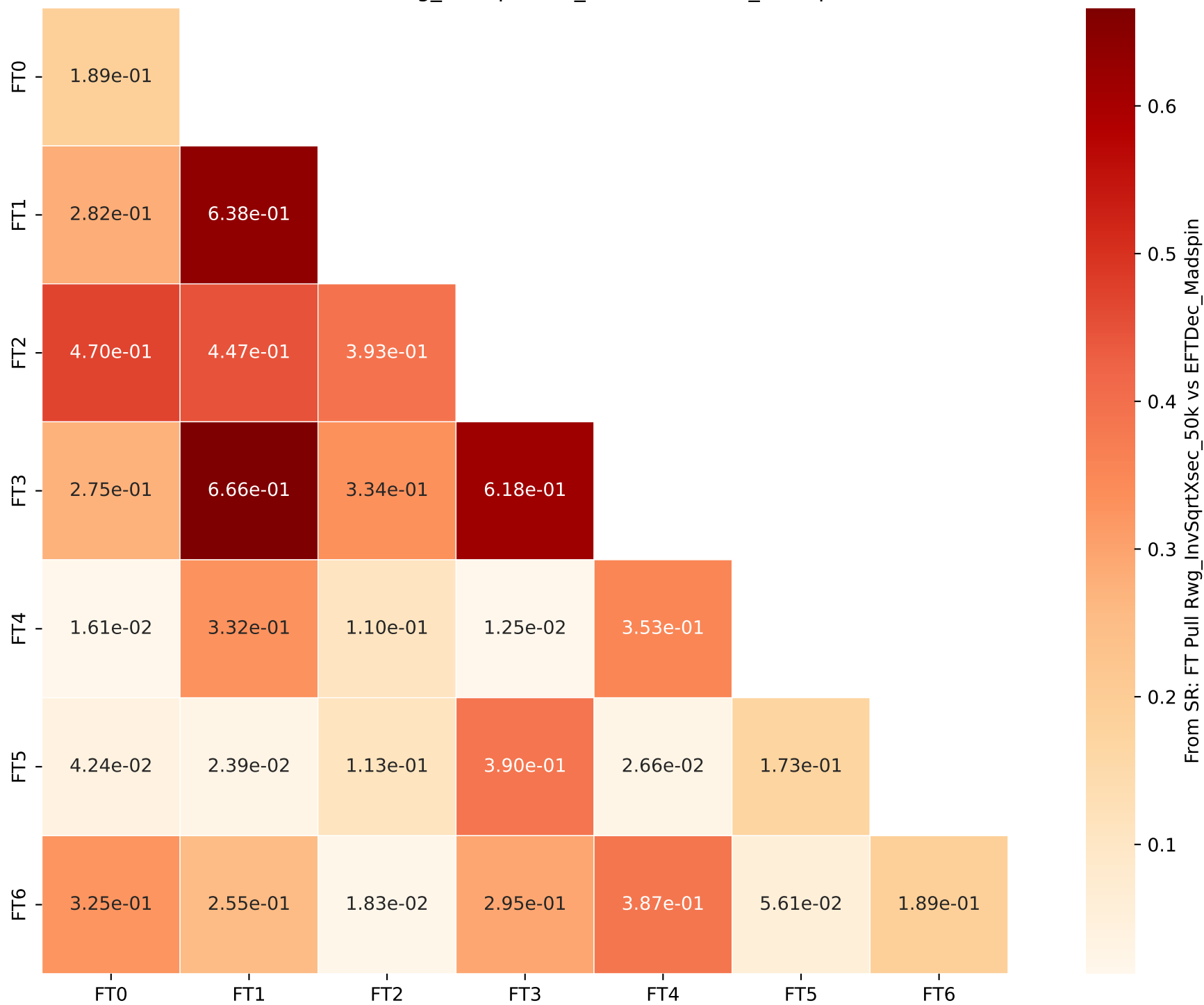
From SR: FT Pull Rwg_InvSqrtXsec_50k vs EFTDec_Madspin
