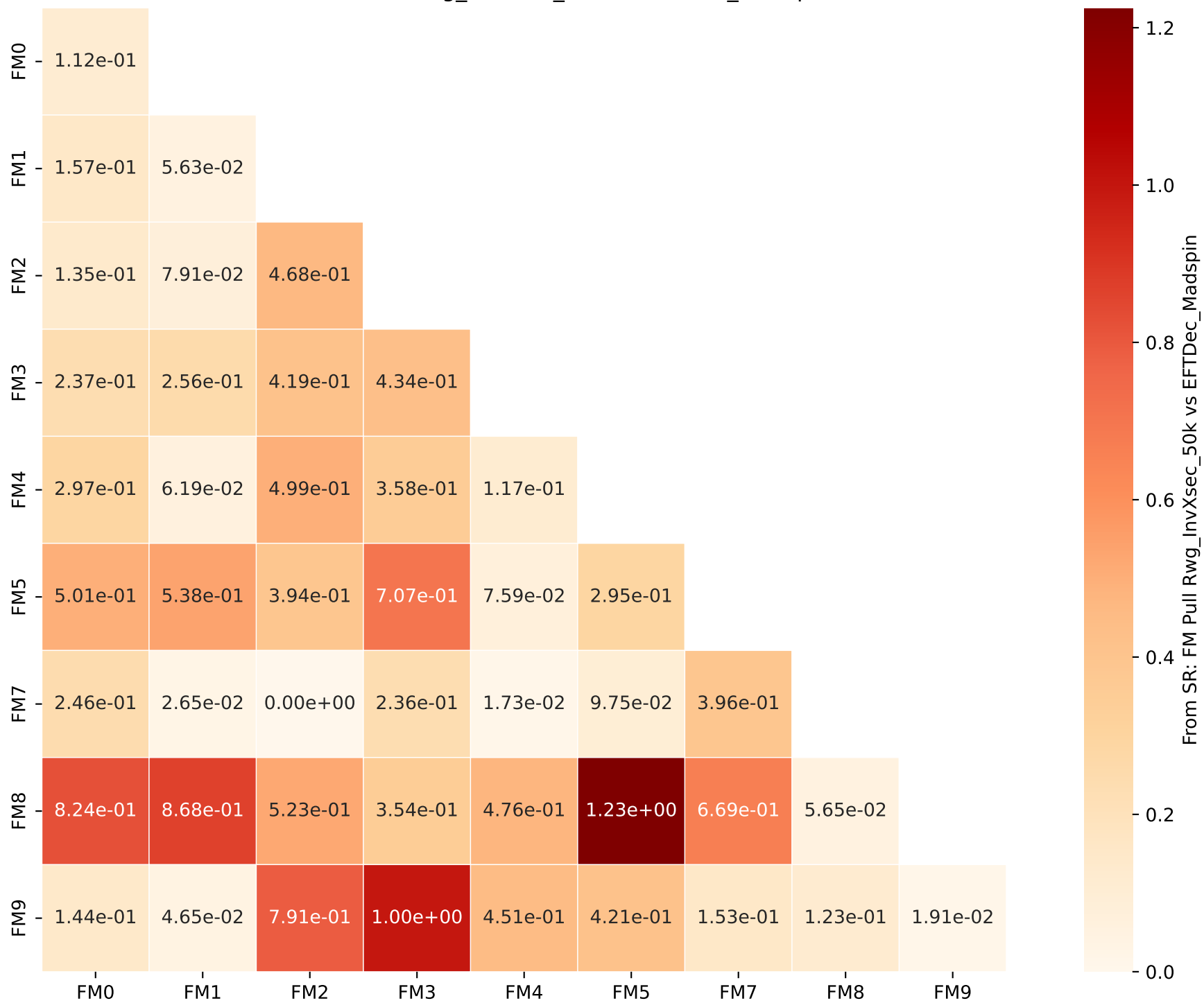
From SR: FM Pull Rwg_InvXsec_50k vs EFTDec_Madspin
