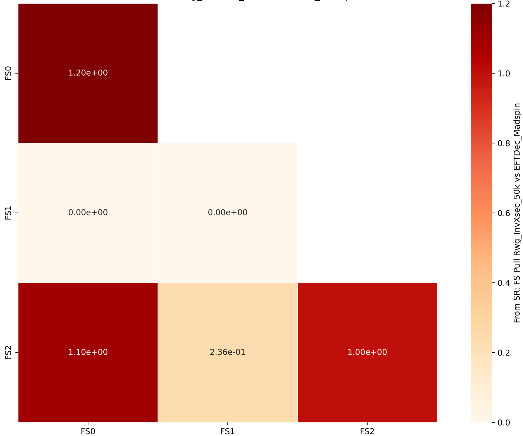
From SR: FS Pull Rwg_InvXsec_50k vs EFTDec_Madspin
