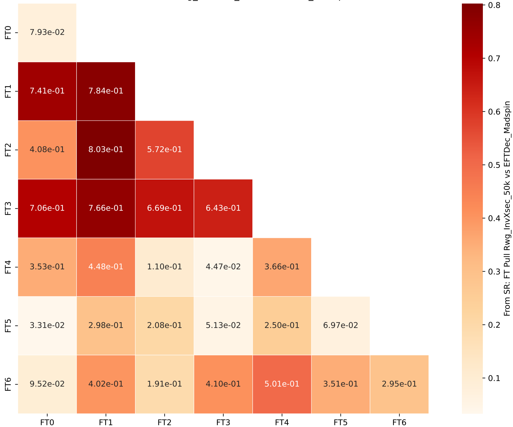
From SR: FT Pull Rwg_InvXsec_50k vs EFTDec_Madspin
