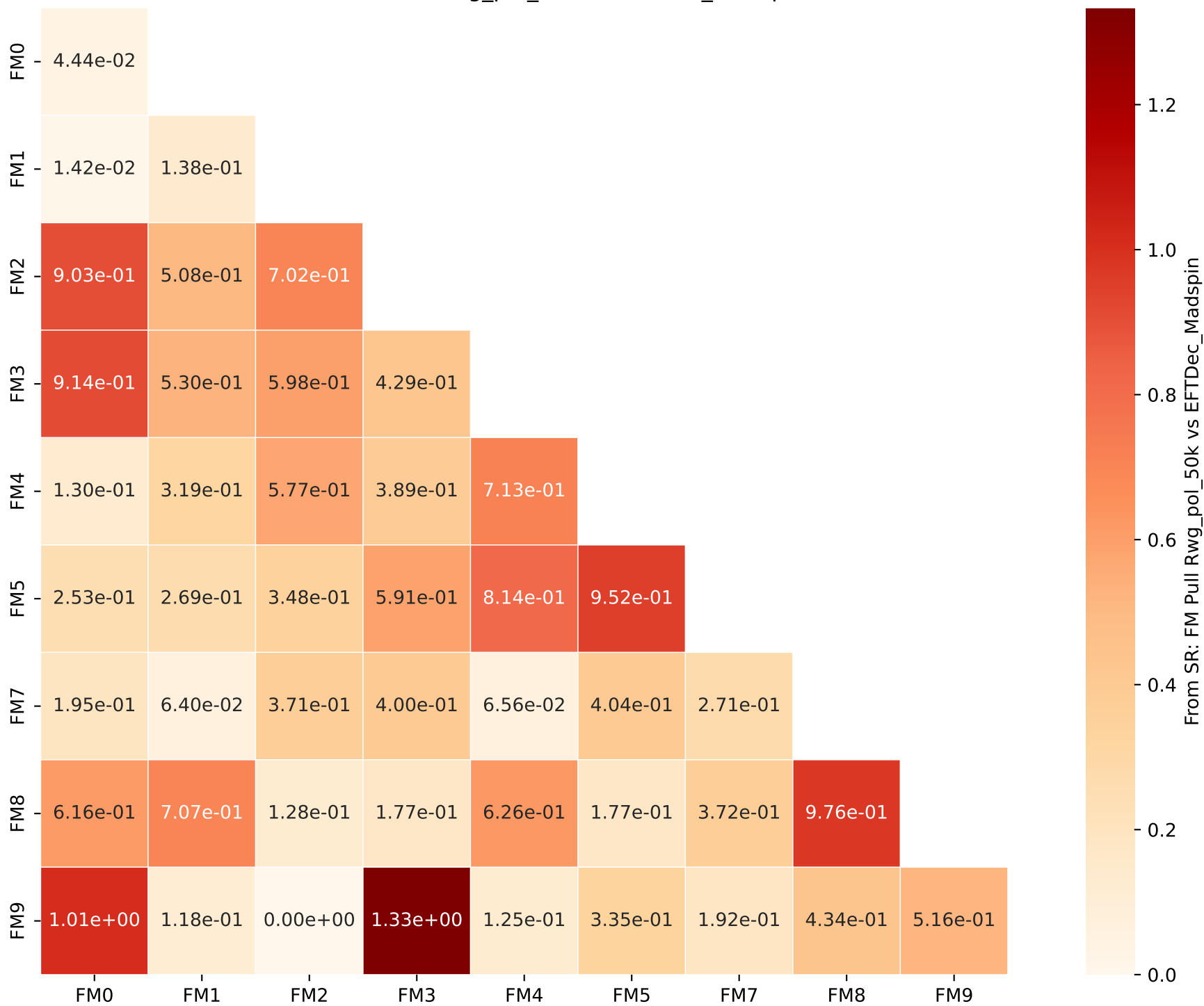
From SR: FM Pull Rwg_pol_50k vs EFTDec_Madspin
