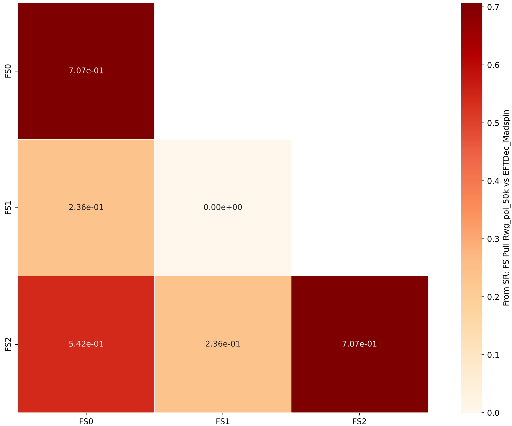
From SR: FS Pull Rwg_pol_50k vs EFTDec_Madspin
