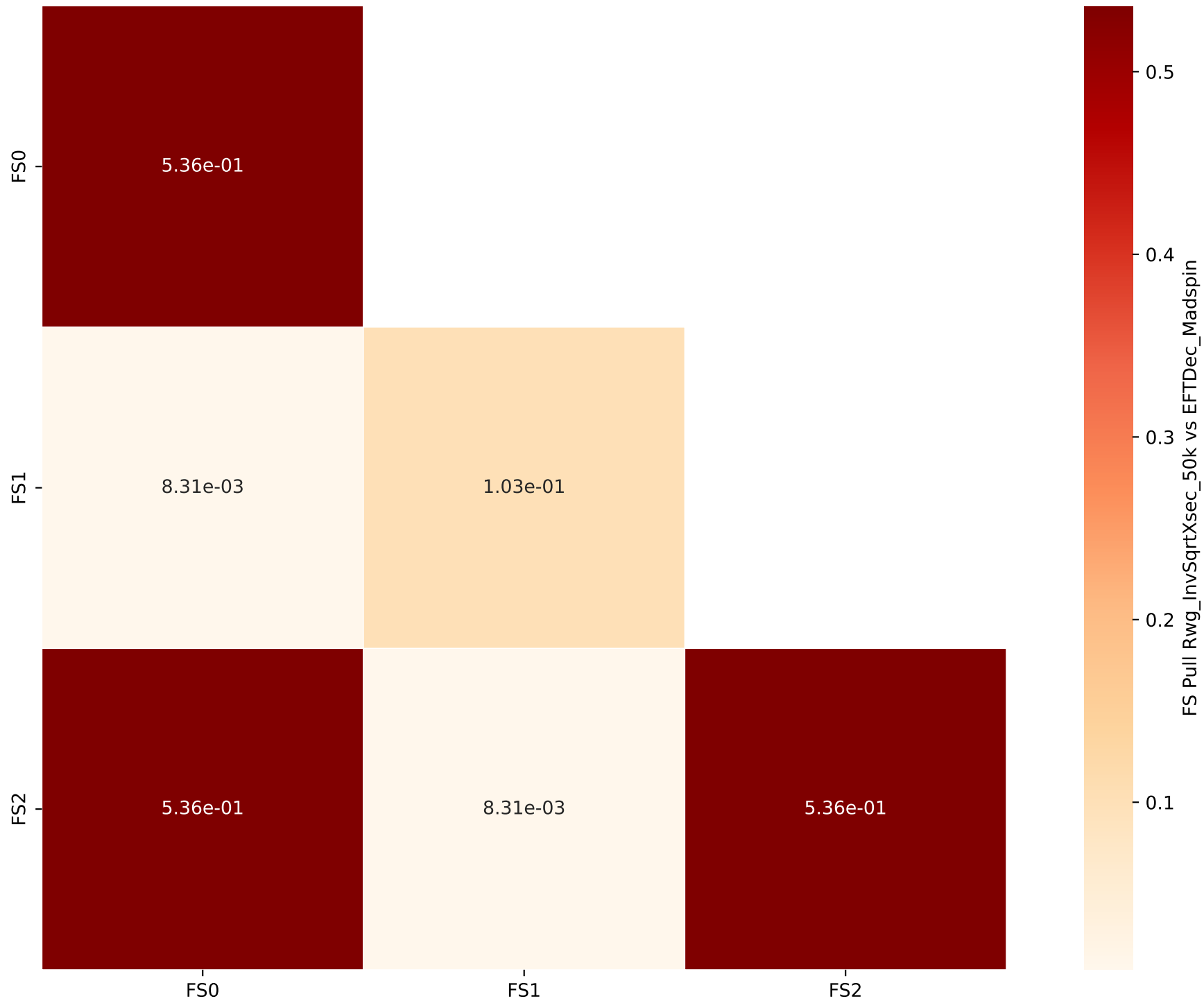
FS Pull Rwg_InvSqrtXsec_50k vs EFTDec_Madspin
