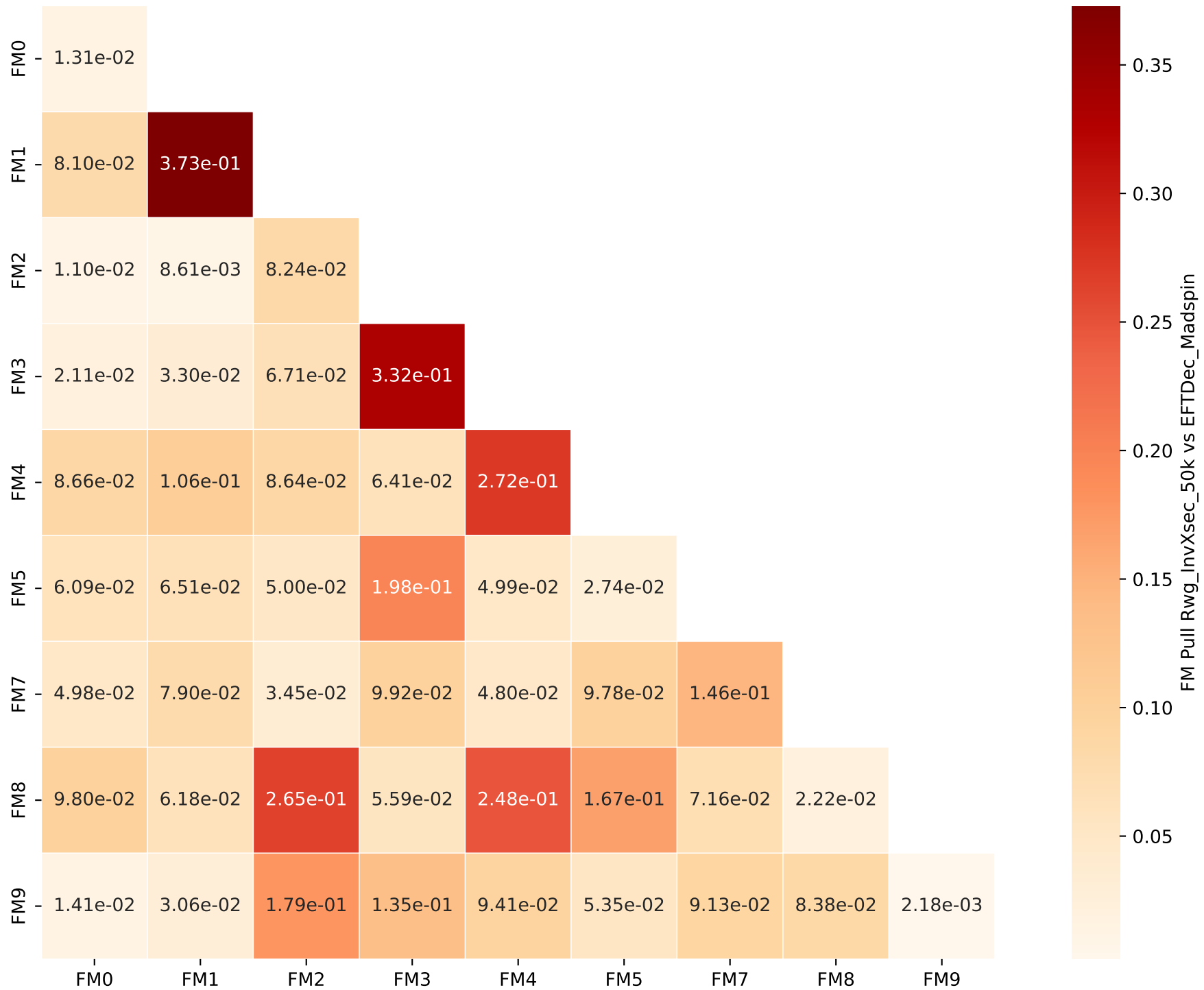
FM Pull Rwg_InvXsec_50k vs EFTDec_Madspin
