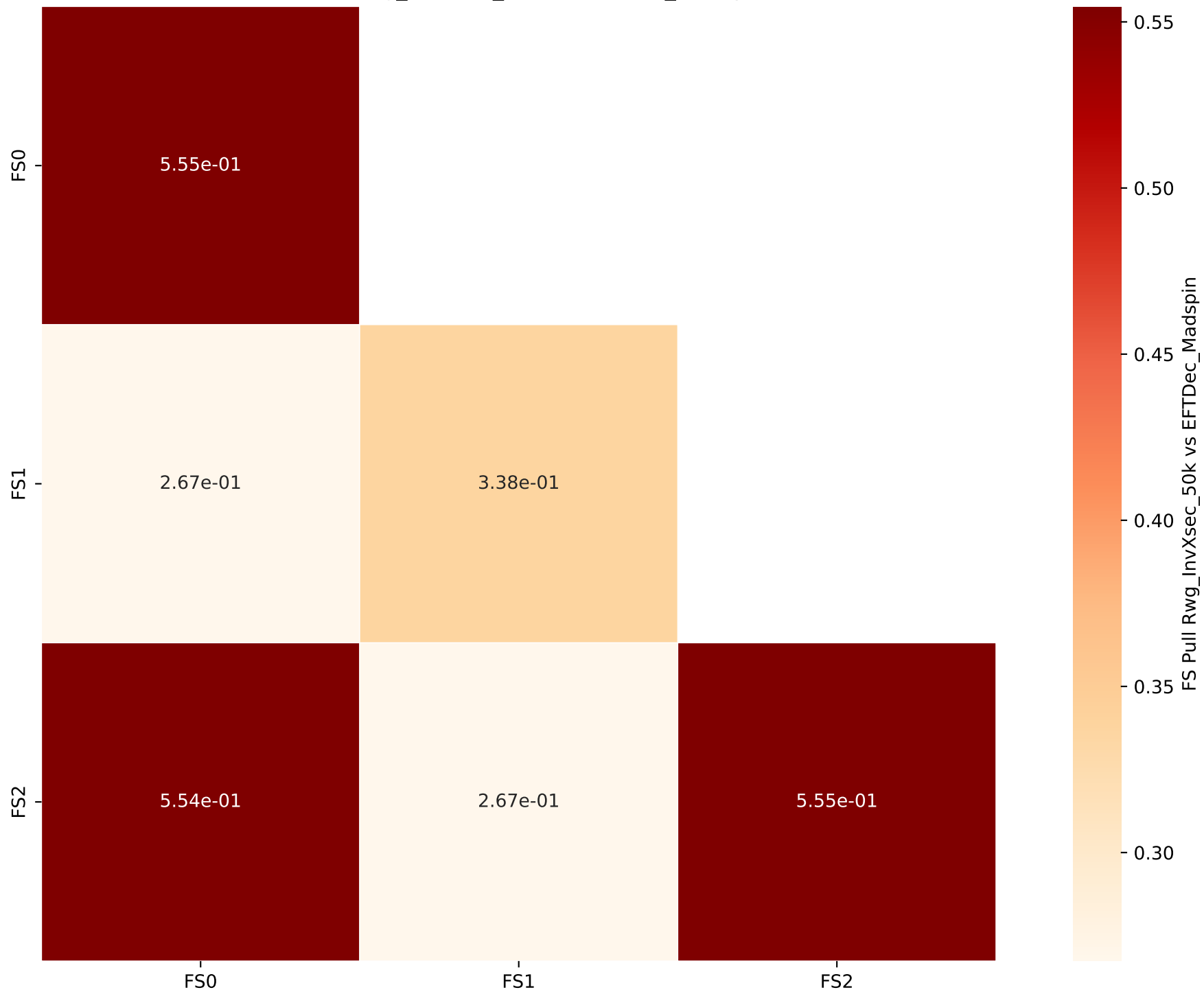
FS Pull Rwg_InvXsec_50k vs EFTDec_Madspin
