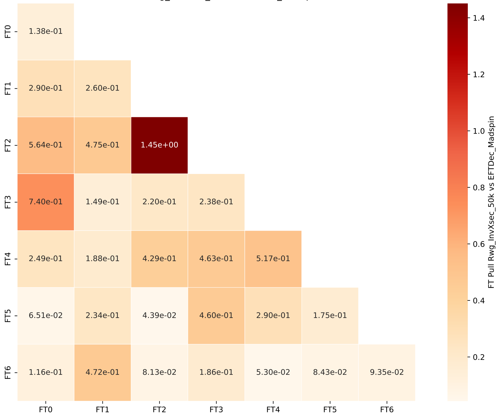
FT Pull Rwg_InvXsec_50k vs EFTDec_Madspin
