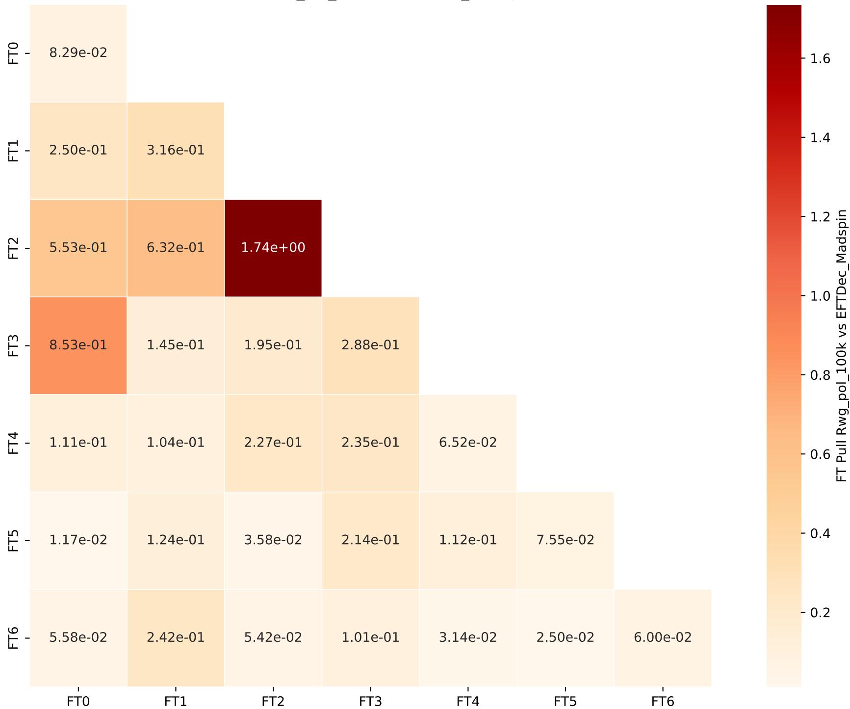
FT Pull Rwg_pol_100k vs EFTDec_Madspin
