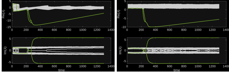
Figura 4: Evolución temporal de la parte real (arriba) e imaginaria (abajo) de los autovalores de W . Se observa como el resultado de la ecuación con la no linealidad \tanh(x) ( Dcha. ) y la linealizada ( Izda. ) no cambia de forma significativa y es cualitativamente idéntica.
