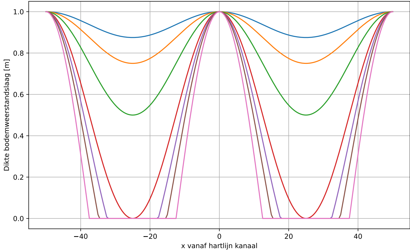
Verloop dikte uitgeschuurde bodemweerstandslaag
