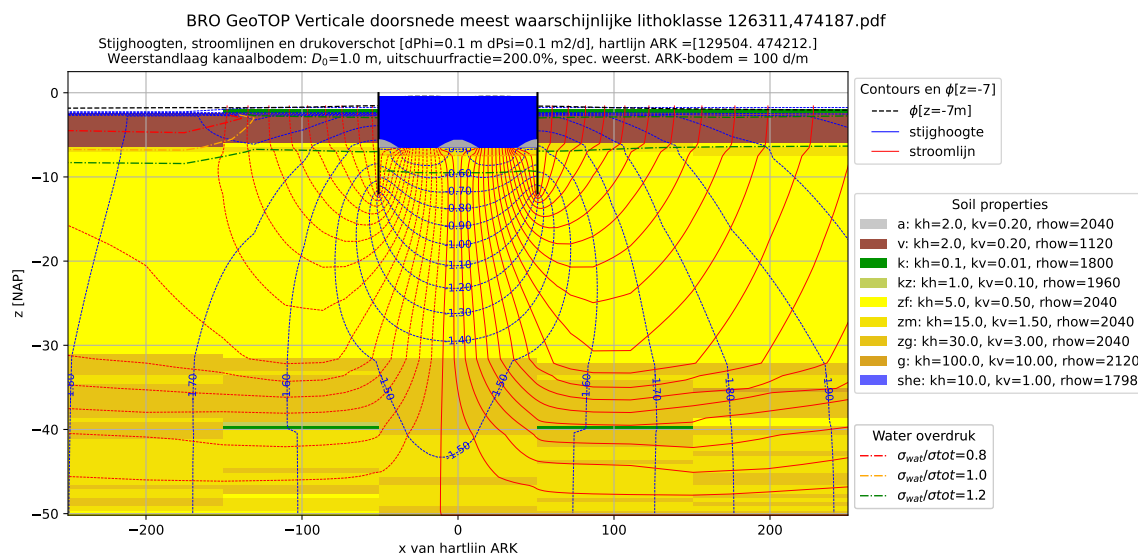
Figuur 13: Situatie waarin de weerstandslaag in de geulen voor 200% is geërodeerd
