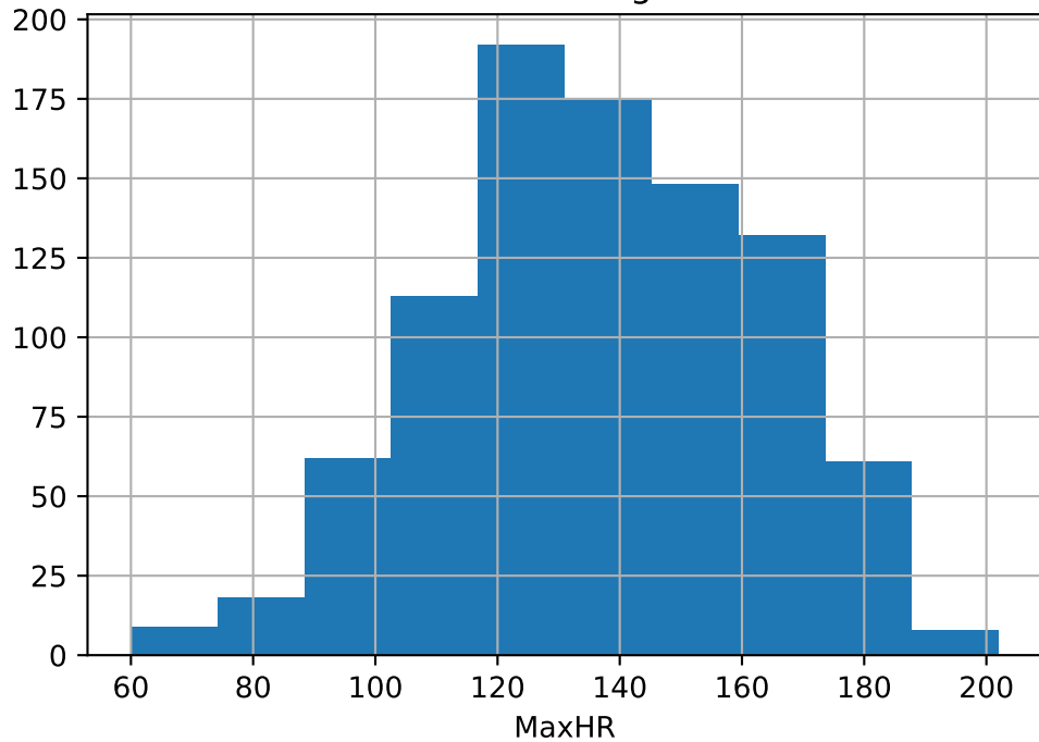
MaxHR Histogram
