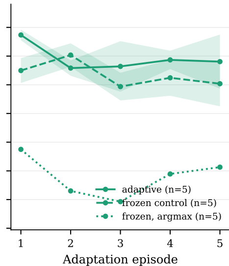
MLP-PPO
