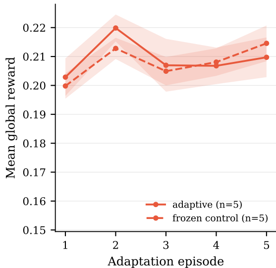
DDQN
