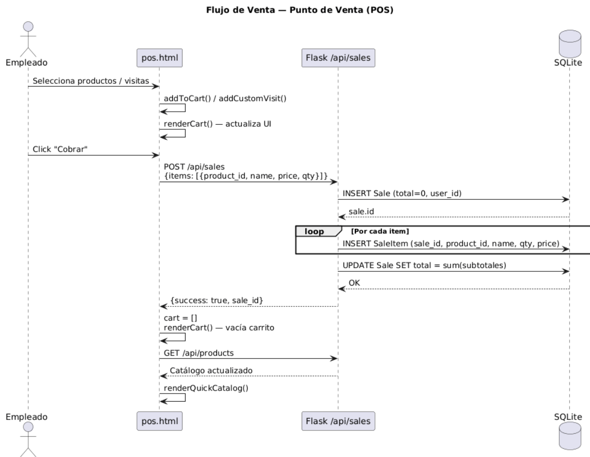
Figura 4. Flujo completo de una venta: desde la selección de productos hasta el commit en la base de datos y descuento de stock.
