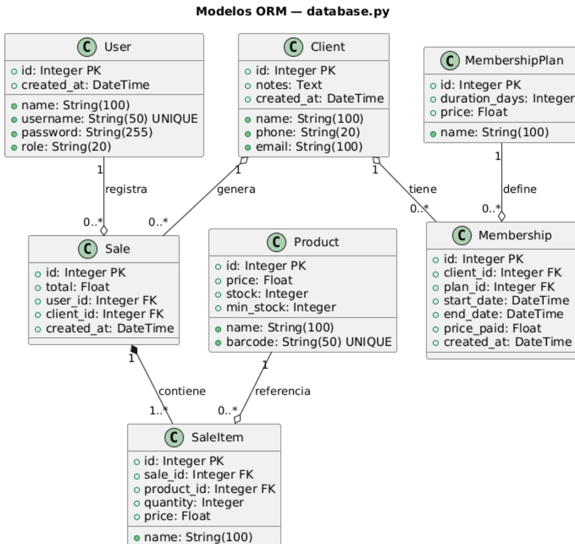
Figura 3. Diagrama de clases ORM — 7 tablas con relaciones de cascada y llaves foráneas indexadas.
