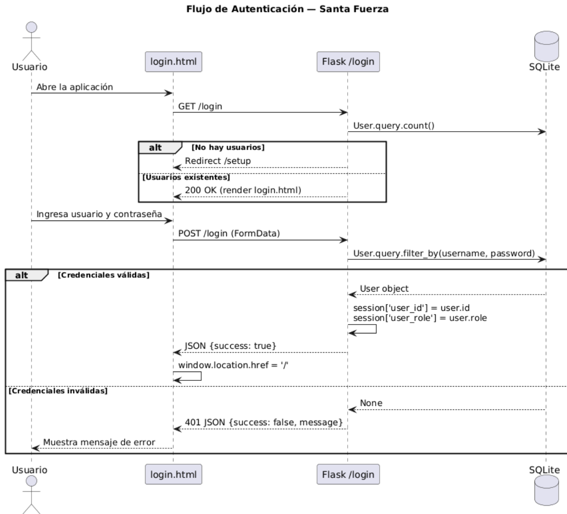
Figura 1. Diagrama de secuencia del proceso de autenticación. El flujo valida credenciales contra la base de datos y establece la sesión RBAC del usuario.
