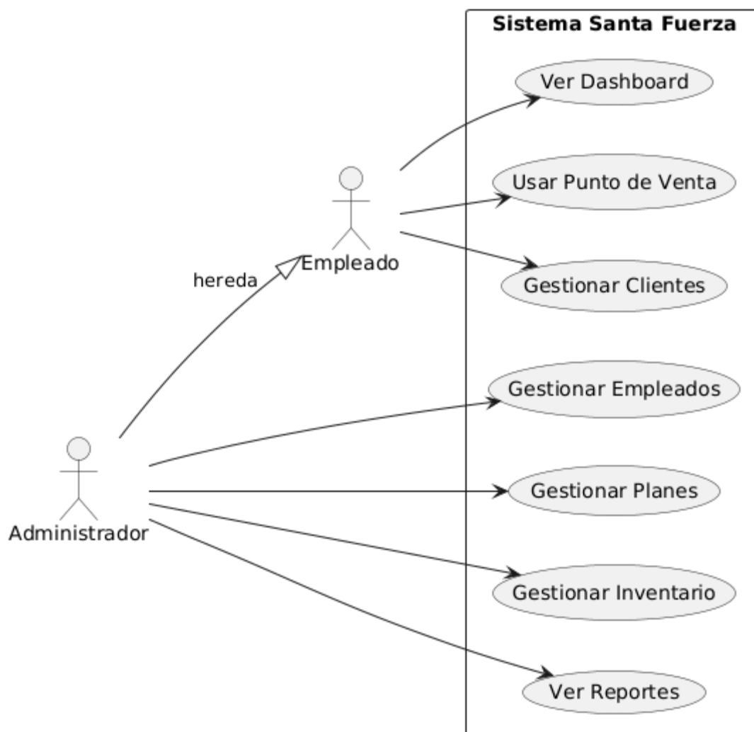
Figura 2. Casos de uso por rol. El rol Admin hereda todas las capacidades del rol Empleado y agrega acceso a módulos de gestión.
