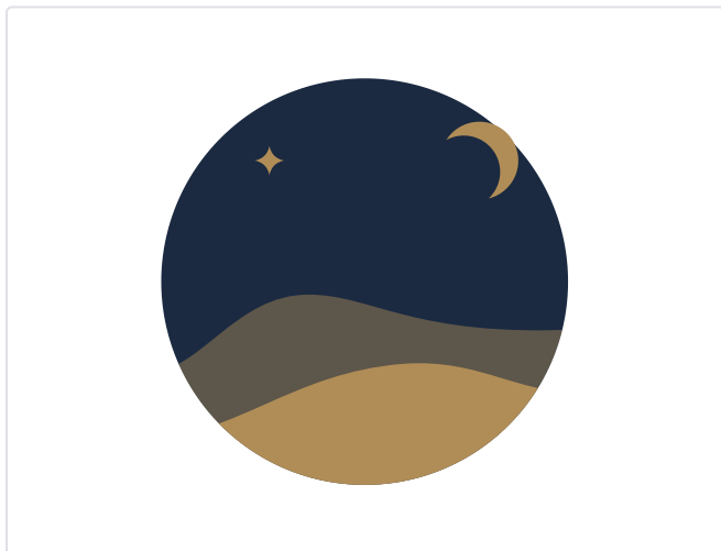
С1 Луна
