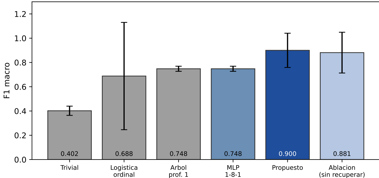
P1: F1 macro, media +- sd entre pliegues (3 semillas)
