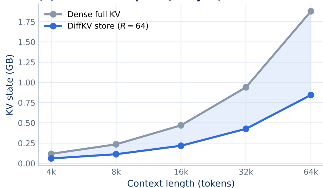
(d) KV-state footprint (analytic)
