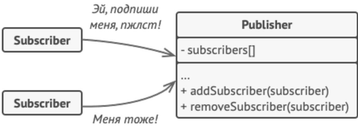
Подписка на события.
