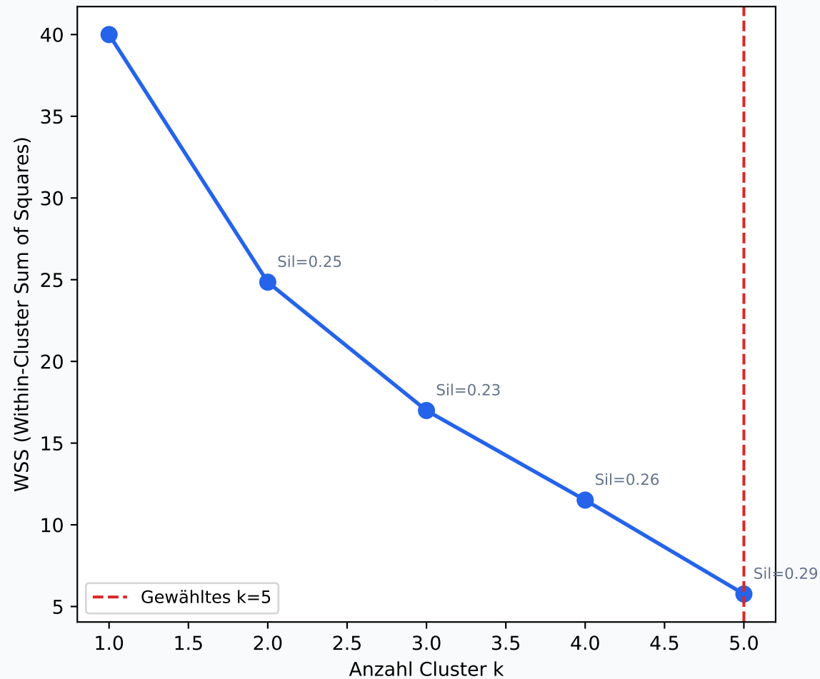
Elbow-Methode (WSS je k)
