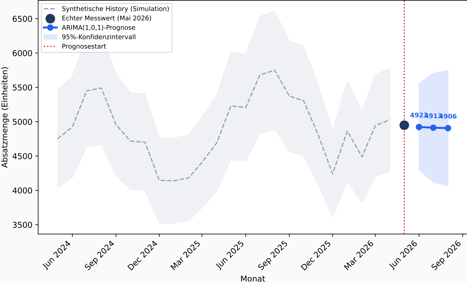
Monatlicher Absatz + 3-Monats-Prognose (Menge in Einheiten)
