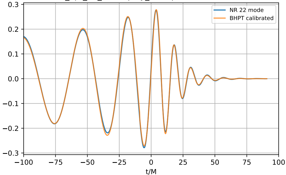
PN_opt_nu_Pade (poly_nu) q=3.0 ; \nu=0.1875
