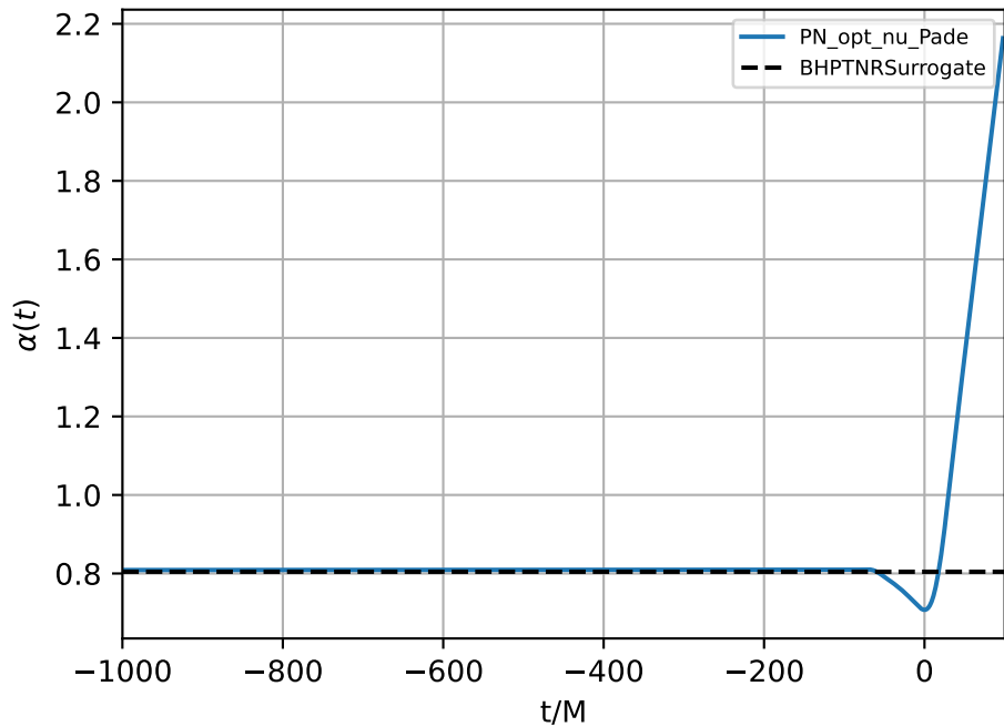
PN_opt_nu_Pade (poly_nu) q=5.0; nu=0.1389
