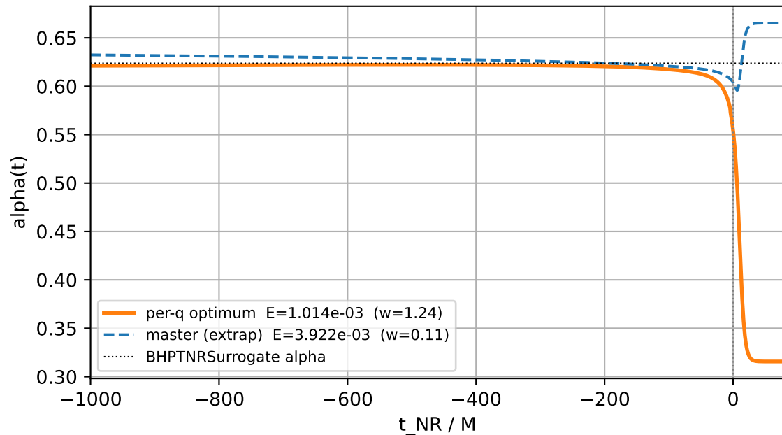
q=2 alpha(t)
