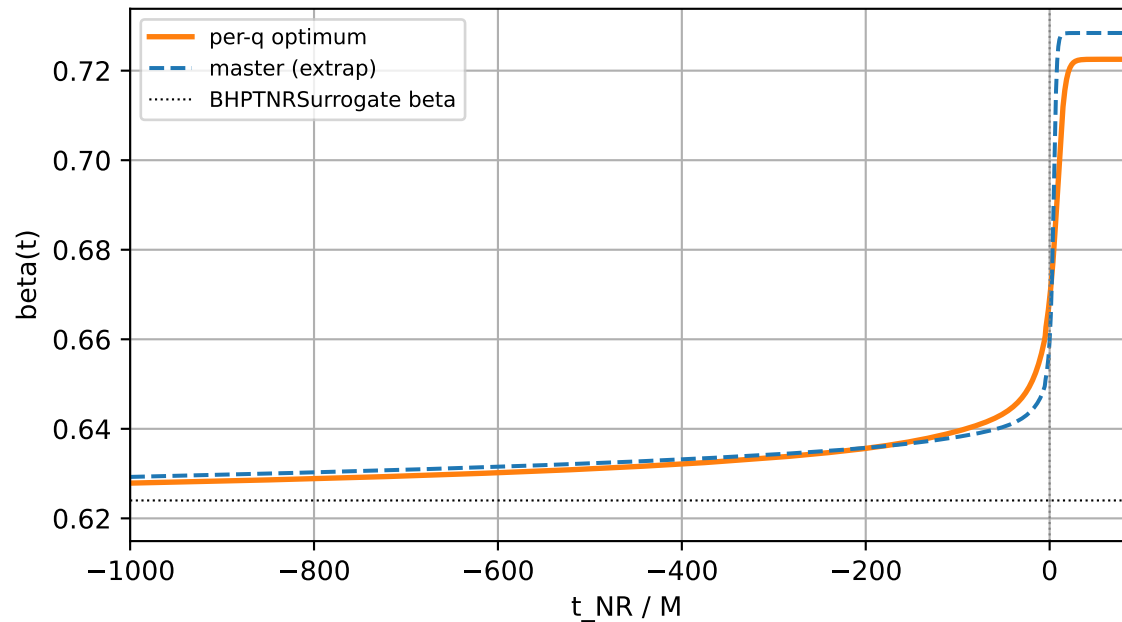
q=2 beta(t)
