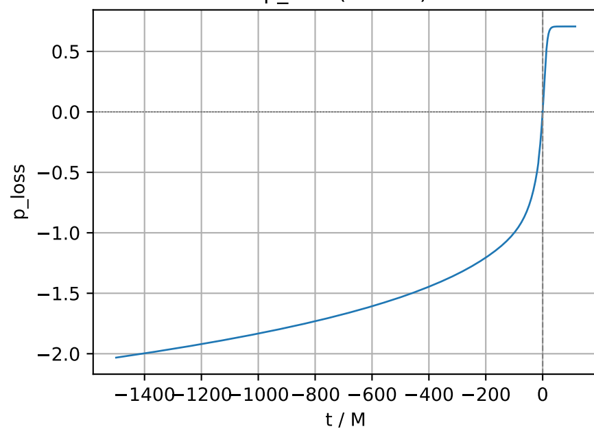
p_{\text{loss}} (wf flux)
