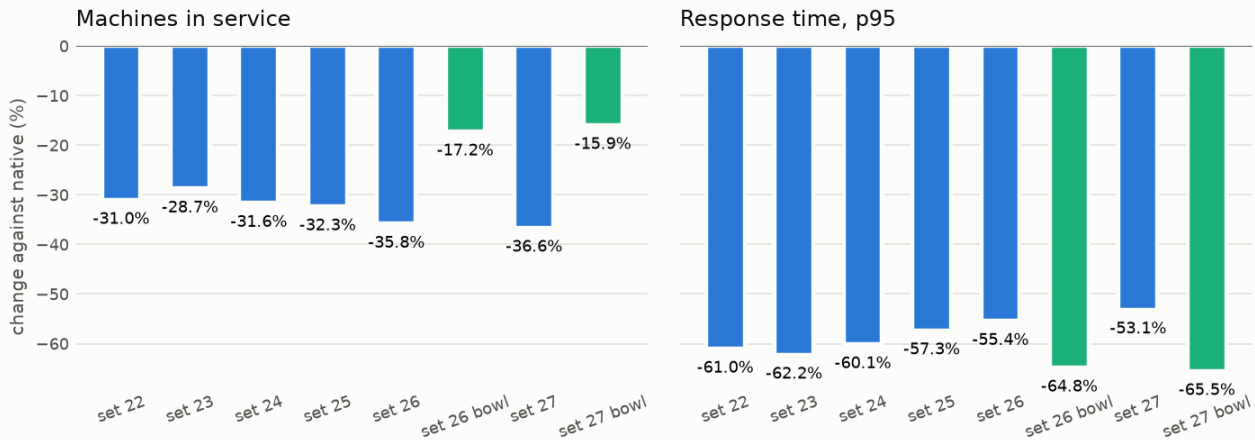
Kubernetes
