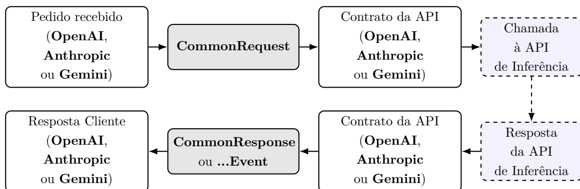
Figura 3.1: Fluxo de normalização entre contratos externos e domínio comum ( OmniAi-SDK )
