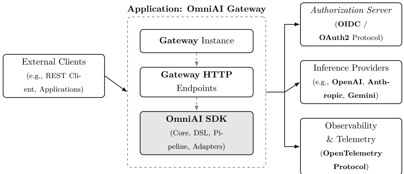
Figura 4.1: Arquitetura Top Level: O OmniAI SDK utilizado para instanciar uma OmniAI Gateway , abstraindo integrações externas padronizadas.
