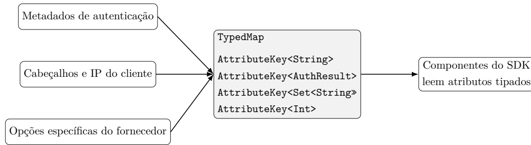
Figura 3.3: Utilização da TypedMap para transportar atributos extensíveis
