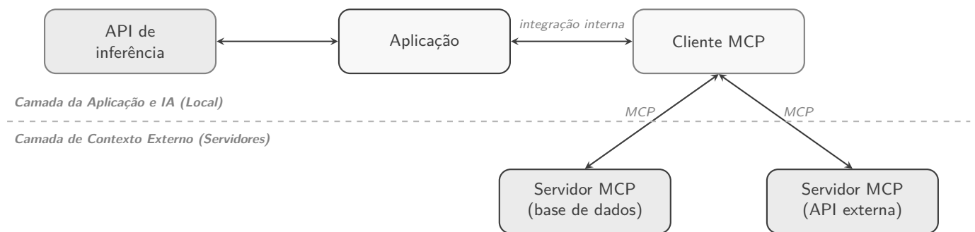
Figura 2.3: Arquitetura simplificada do MCP: separação entre a API de inferência, a aplicação com cliente MCP integrado e a comunicação com servidores externos.
