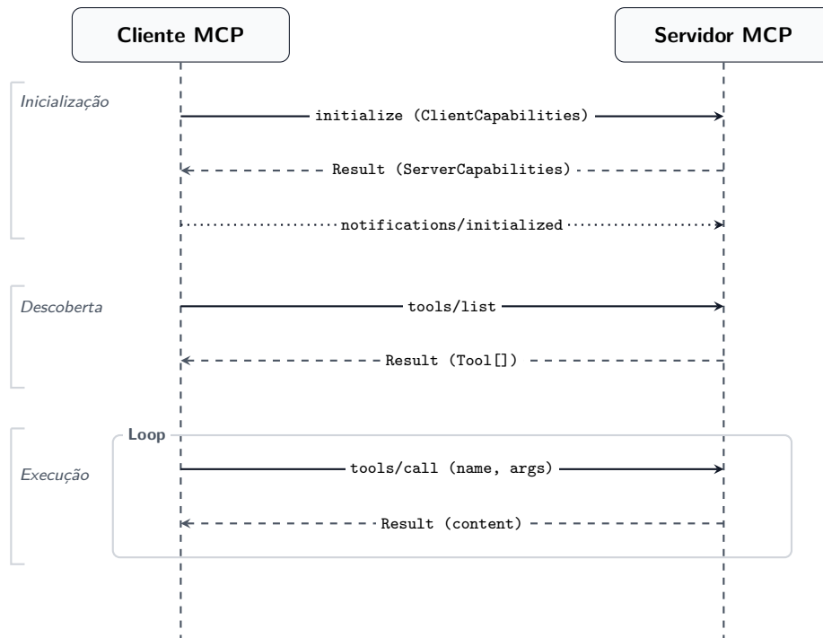
Figura 2.4: Fluxo de comunicação MCP: inicialização por handshake JSON-RPC, descoberta de capacidades e execução de ferramentas.
