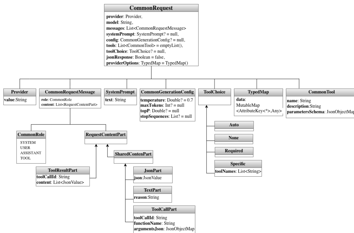
Figura 3.4: Estrutura de classes do CommonRequest .
