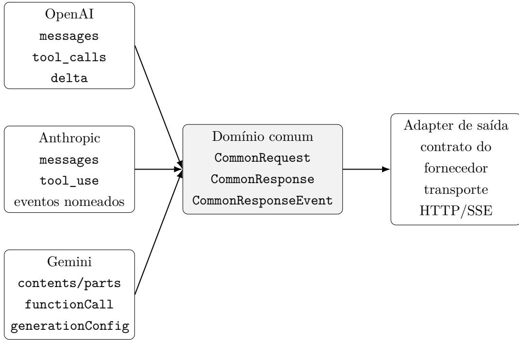
Figura 2.1: Normalização dos contratos de inferência para um domínio comum
