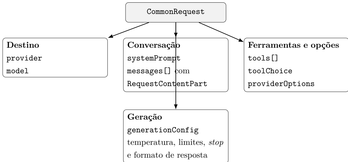
Figura 3.2: Estrutura interna principal de CommonRequest
