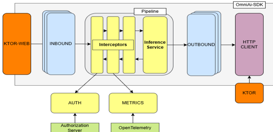
Figura 4.2: Visão da integração entre Ktor, inbounds, pipeline, interceptors, outbounds e HTTP client no OmniAI SDK
