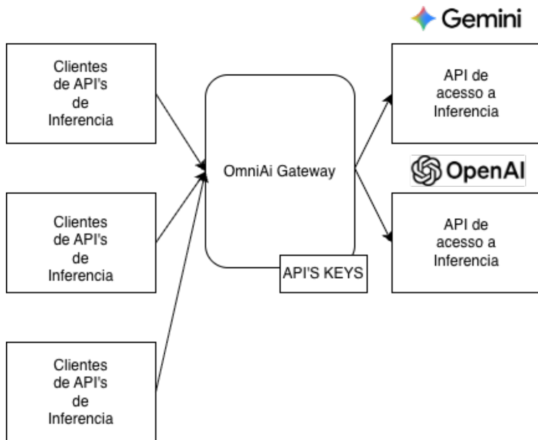
Figura 1.4: Centralização com OmniAI Gateway
