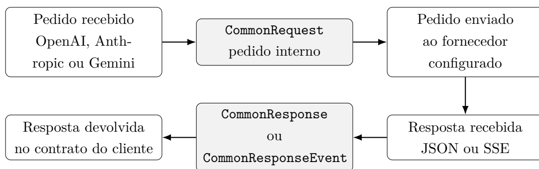
Figura 3.1: Fluxo de normalização entre contratos externos e domínio comum
