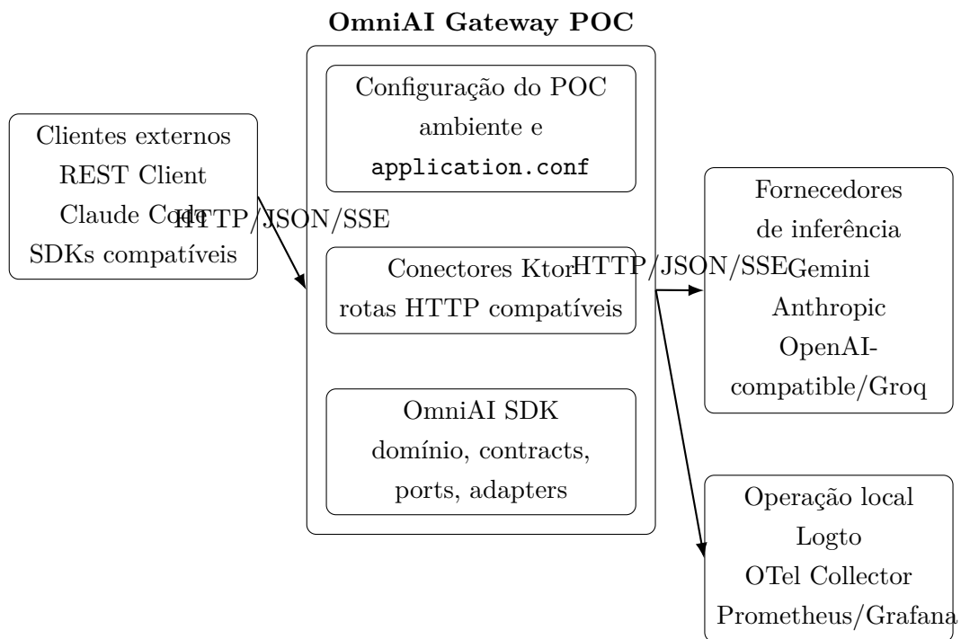
Figura 4.1: Arquitetura top-level: POC OmniAI Gateway a instanciar e demonstrar o OmniAI SDK
