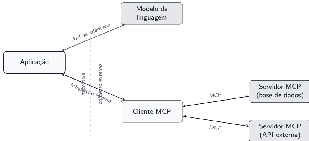
Figura 2.3: Arquitetura do MCP: separação entre a camada de inferência (API do modelo) e a camada de contexto externo (servidores MCP).
