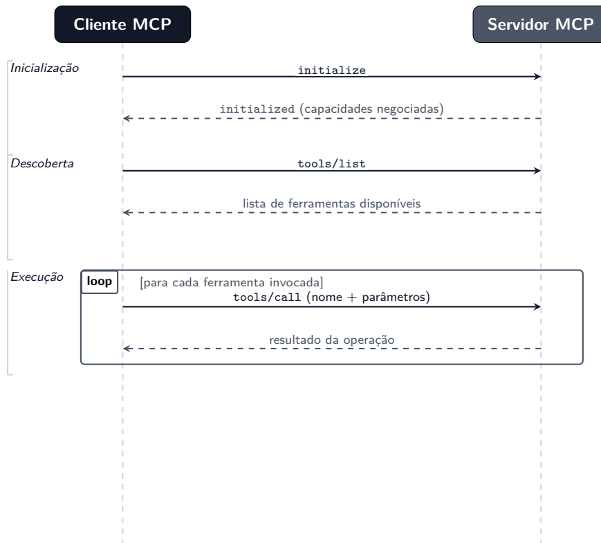
Figura 2.5: Sequência de comunicação MCP: inicialização da sessão, descoberta de capacidades e execução de ferramentas via JSON-RPC.
