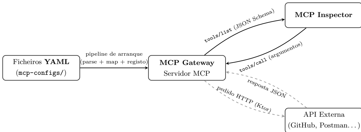
Figura 6.1: Visão geral da MCP Gateway: registo de ferramentas via YAML e execução de pedidos HTTP a APIs externas.
