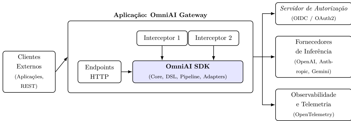
Figura 4.1: Arquitetura de Alto Nível: O OmniAI SDK utilizado para instanciar uma OmniAI Gateway , abstraindo integrações externas padronizadas.
