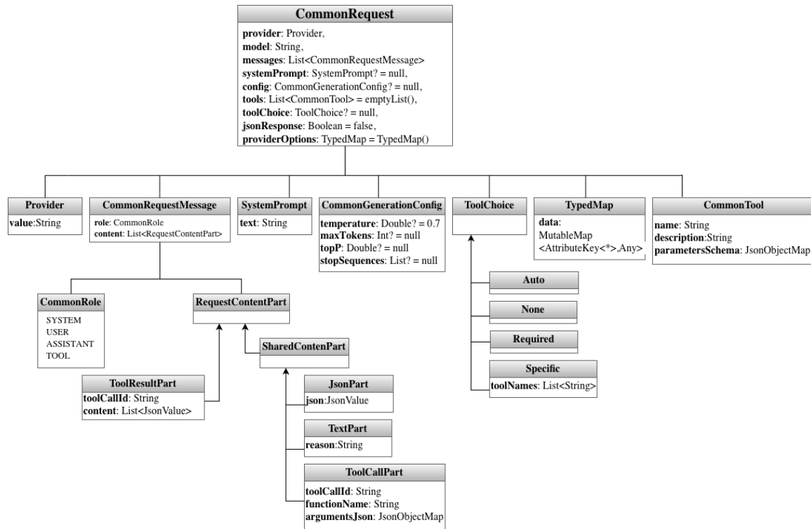
Figura 3.2: Estrutura de classes do CommonRequest .
