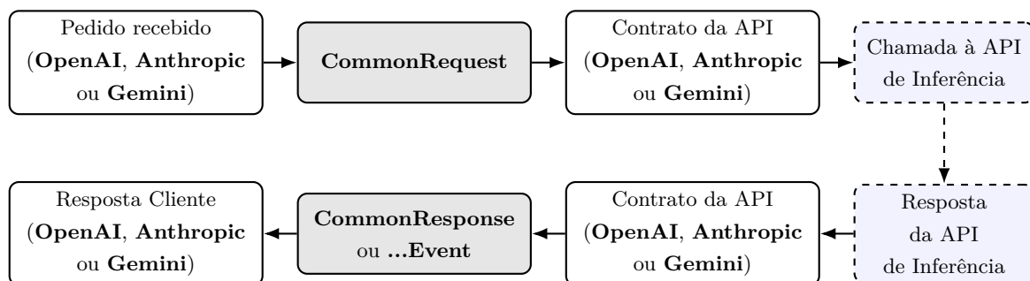
Figura 3.1: Fluxo de normalização entre contratos externos e domínio comum ( OmniAI-SDK )
