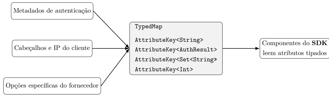
Figura 3.4: Utilização da TypedMap para transportar atributos extensíveis
