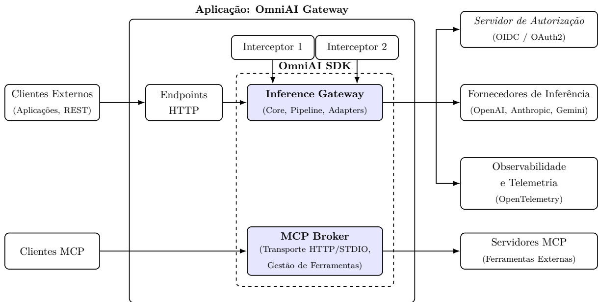
Figura 3.1: Arquitetura de Alto Nível: O OmniAI SDK utilizado para instanciar uma OmniAI Gateway , com a Inference Gateway a abstrair integrações externas padronizadas e o MCP Broker a gerir ferramentas.
