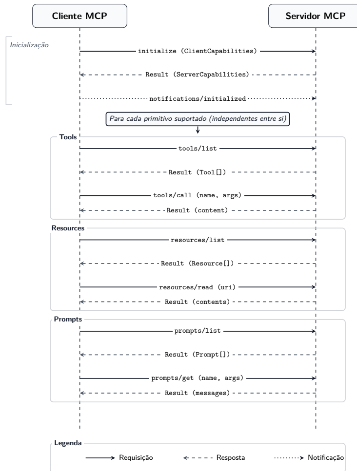
Figura 2.4: Fluxo de comunicação MCP - Adaptado da Documentação do MCP [12]
