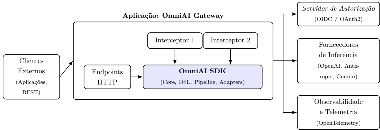
Figura 3.1: Arquitetura de Alto Nível: O OmniAI SDK utilizado para instanciar uma OmniAI Gateway , abstraindo integrações externas padronizadas.
