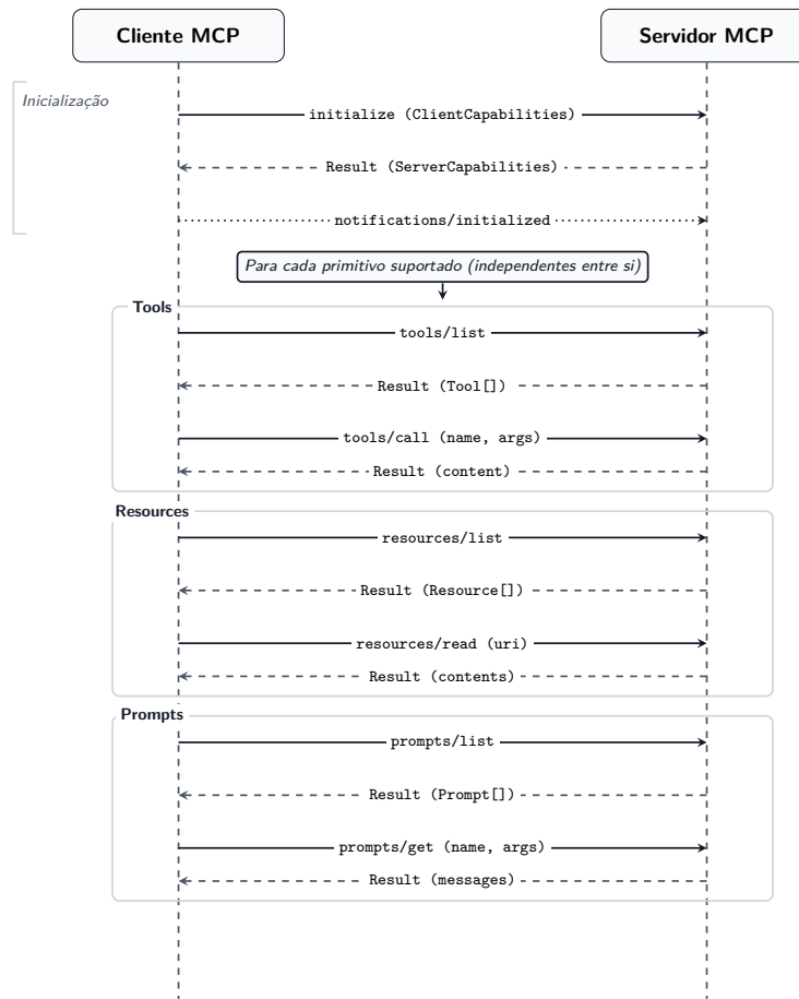
Figura 2.4: Fluxo de comunicação MCP: inicialização por handshake JSON-RPC, seguida da descoberta e invocação de cada tipo de primitivo ( tools , resources e prompts ). Estes três blocos partilham a mesma sessão e podem ser exercidos pelo cliente em qualquer ordem, consoante as capacidades anunciadas pelo servidor na fase de inicialização.
