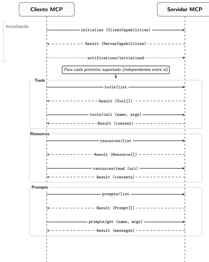
Figura 2.4: Fluxo de comunicação MCP - Adaptado da Documentação do MCP [?]
