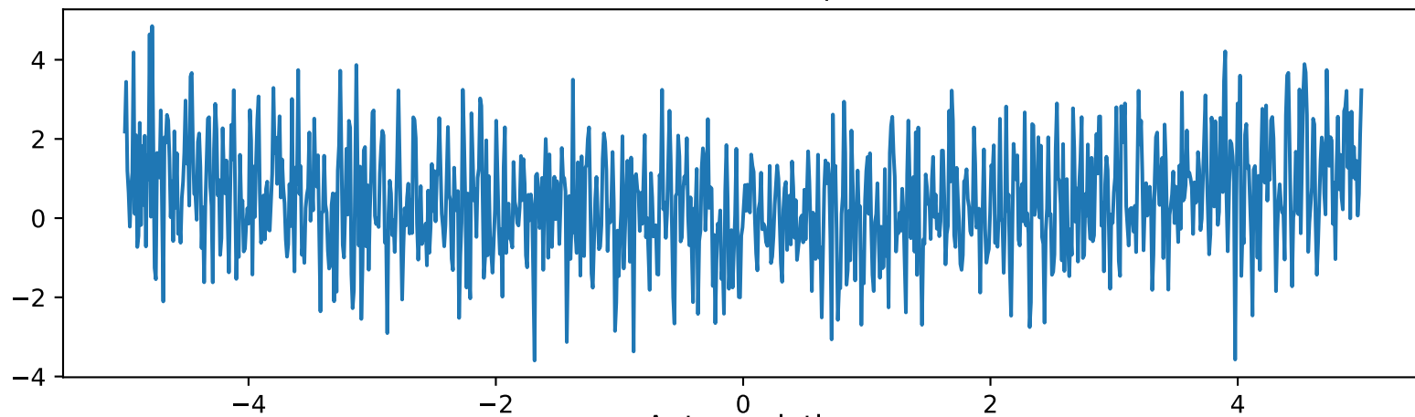
Autocorelatia
