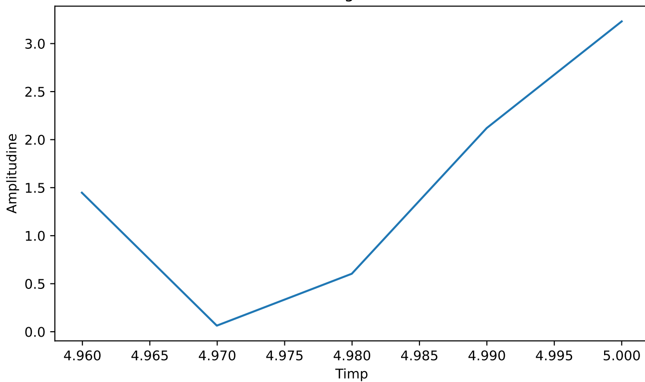
Predictie (m=50, p=39)
