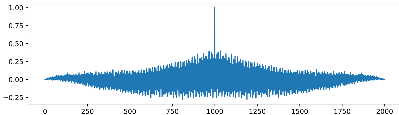
Autocorelatia
