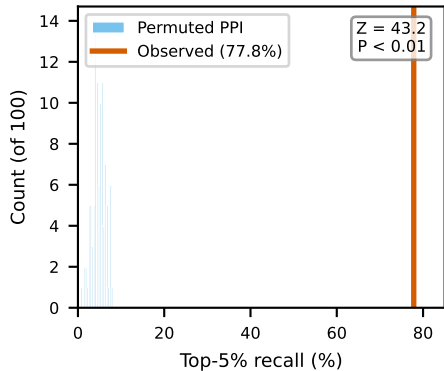
Set 1 (n = 167)
