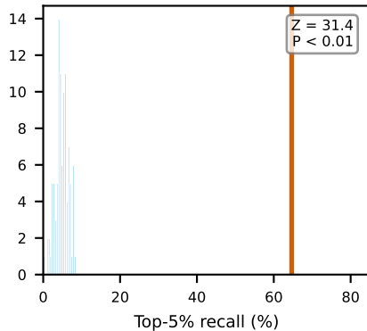
Set 2 (n = 133)
