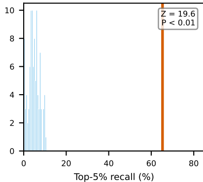
Set 3 (n = 49)
