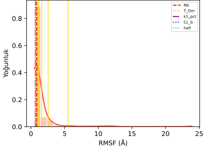
R2 KDE | Tüm UST sınırları
