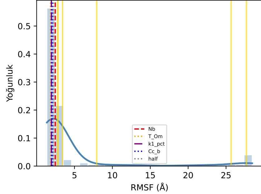
R1 KDE | Tüm UST sınırları
