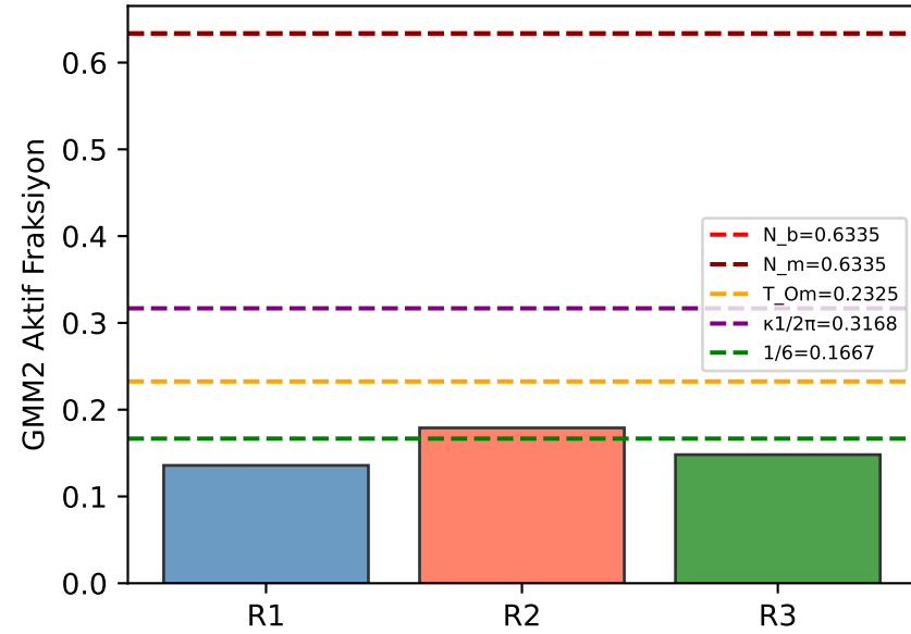
Aktif fraksiyon vs tüm UST sabitleri
