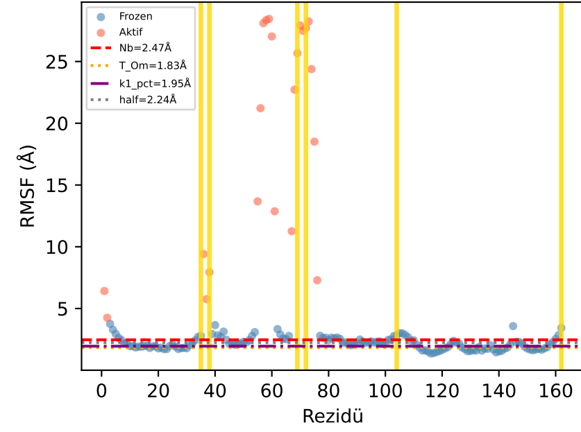
R1 | ort=4.464Å Aktif=0.1358 CxxC/g=2.627
