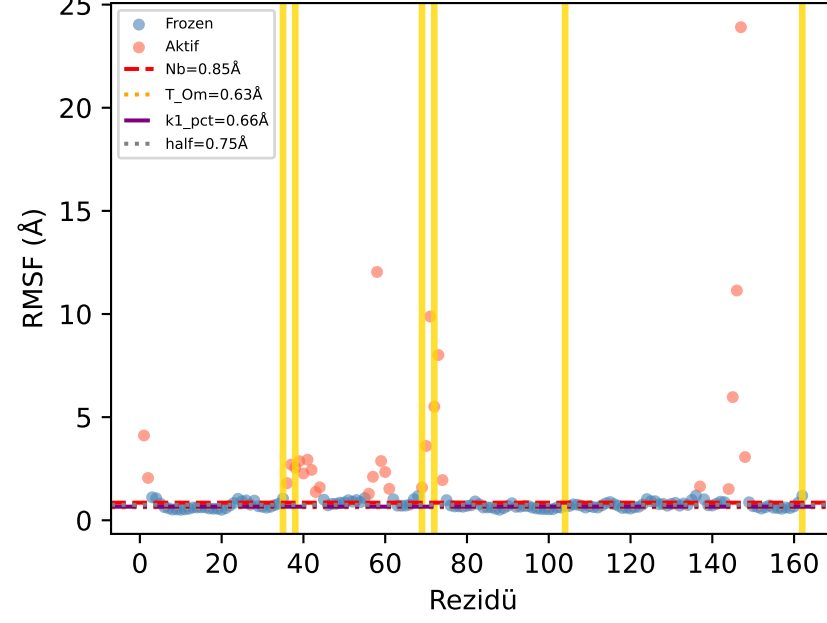
R2 | ort=1.391Å Aktif=0.1790 CxxC/g=1.509
