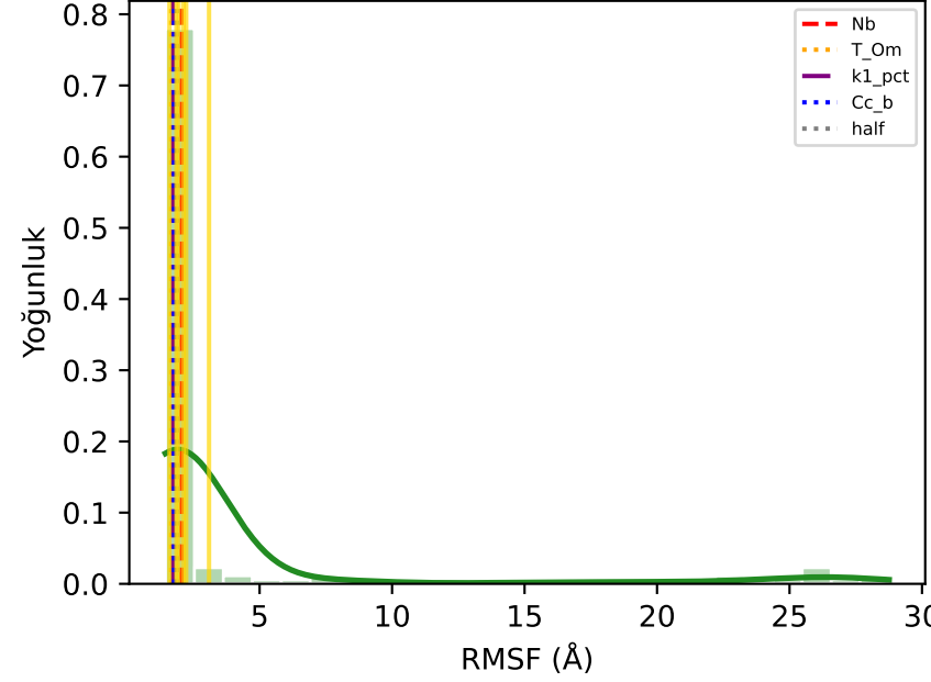
R3 KDE | Tüm UST sınırları
