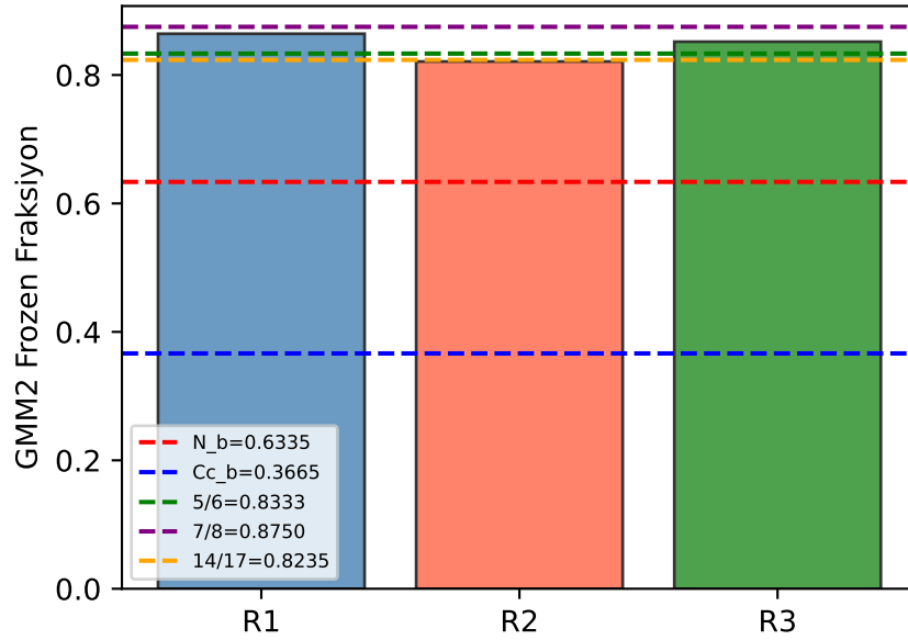
Frozen fraksiyon vs tüm UST sabitleri
