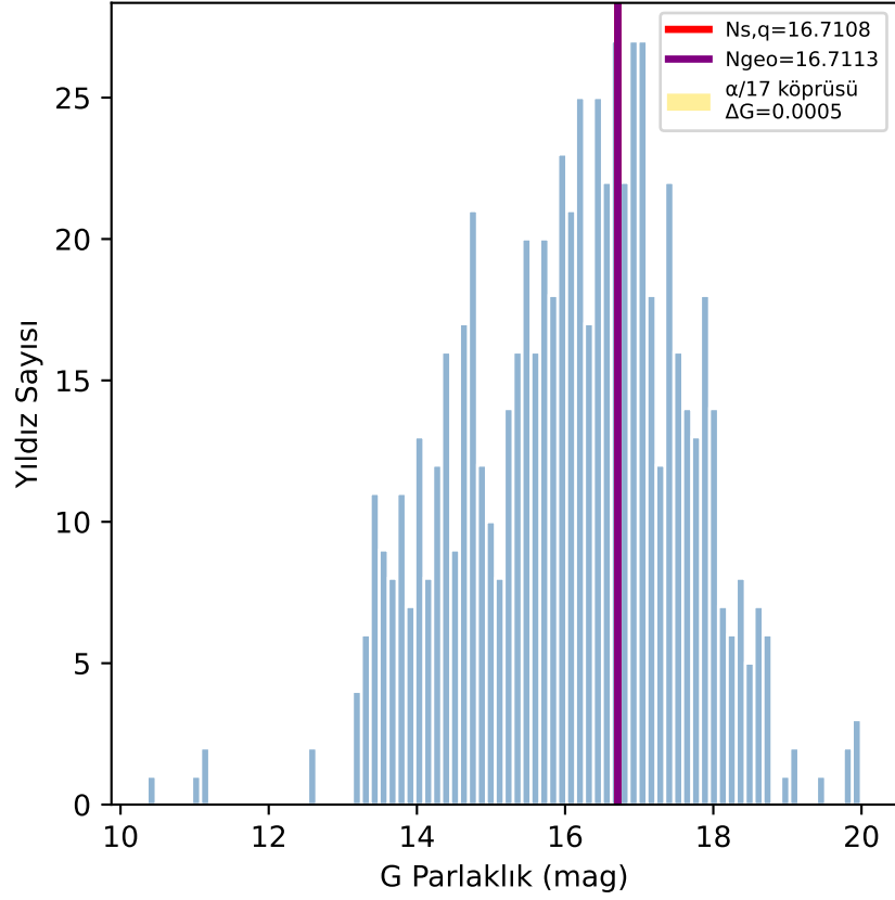
α/17 Omnium Köprüsü Ngeo → Ns,q Geçiş Bölgesi
