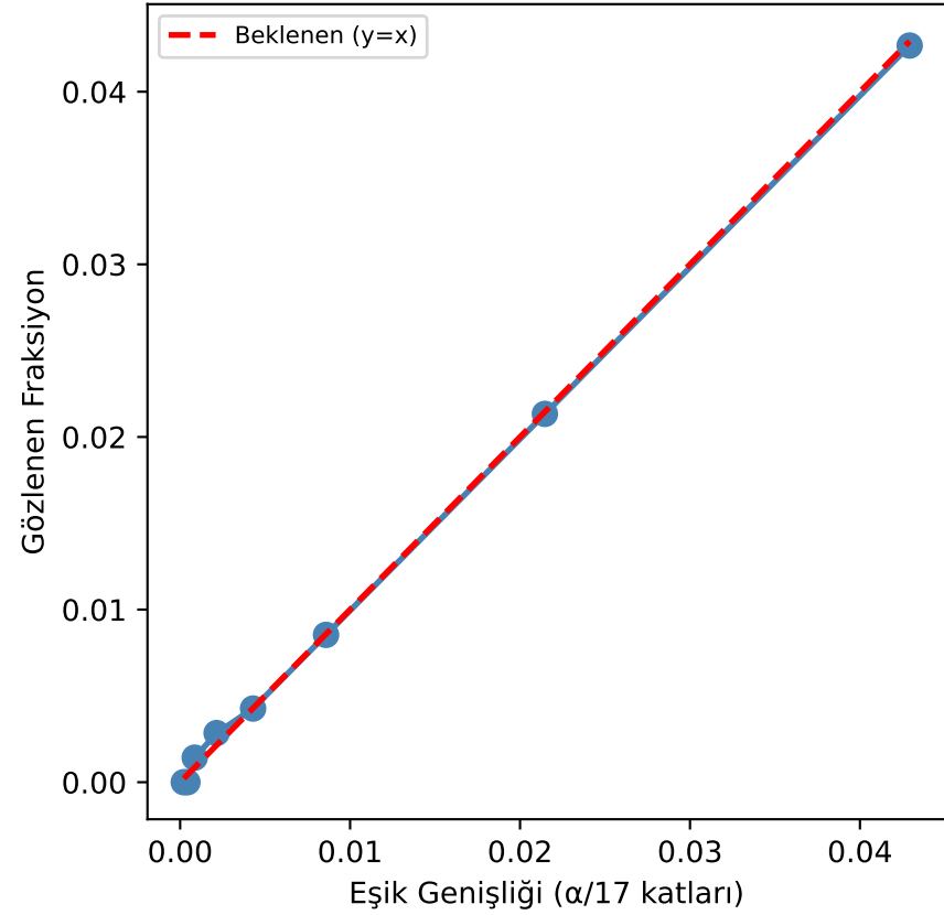
α/17 Eşik Genişliği Testi
