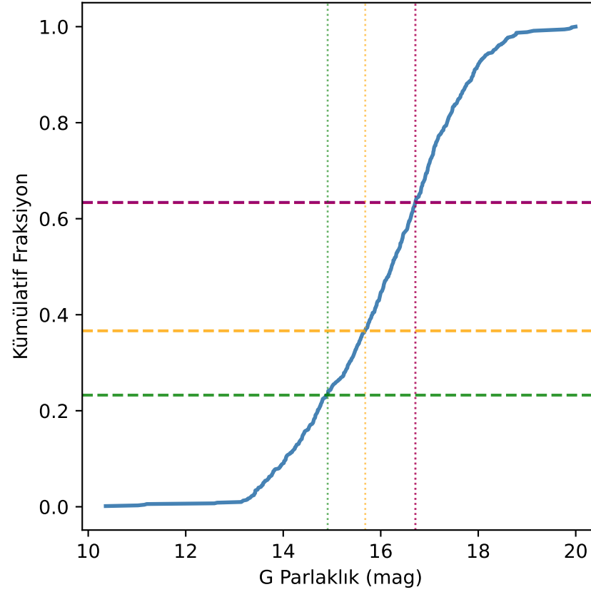
CDF + UST Sınırları Ns,q, Ngeo, T0m, Ccb
