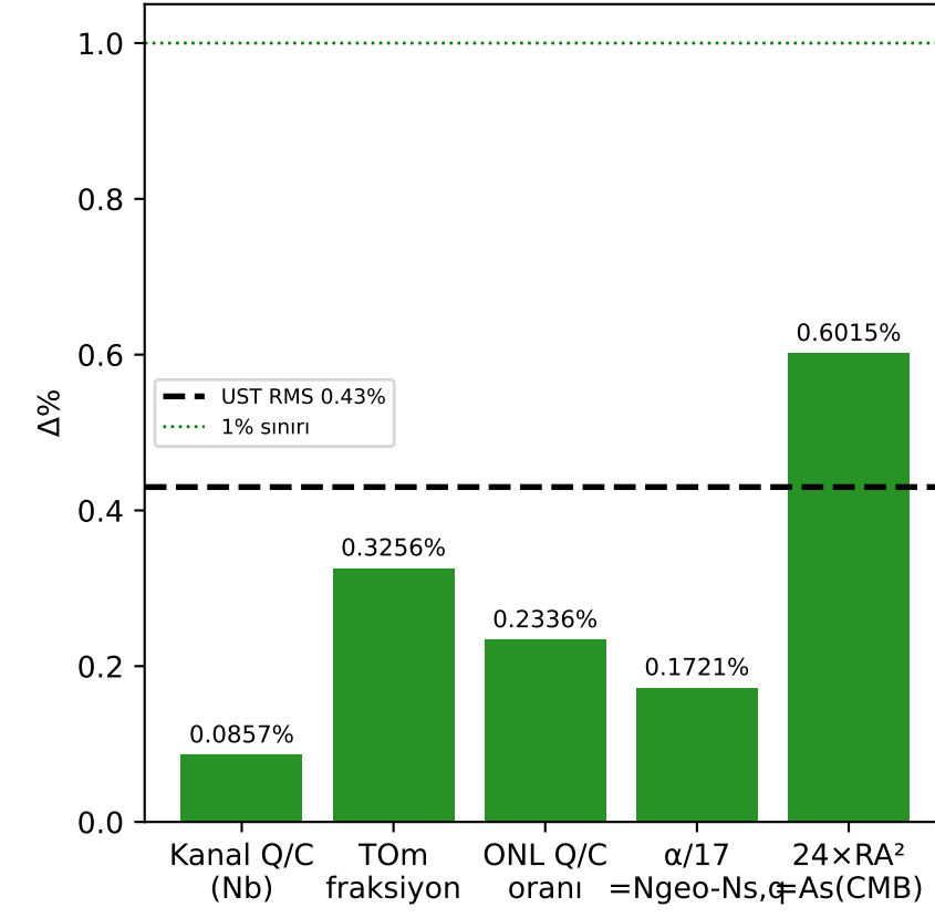
UST Tam Test Skoru (RA 2 ve α/17 dahil)
