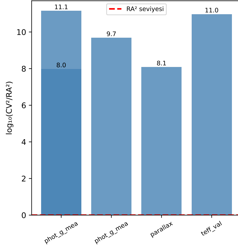
RA 2 Varyans Analizi CV 2 /RA 2 log oranları
